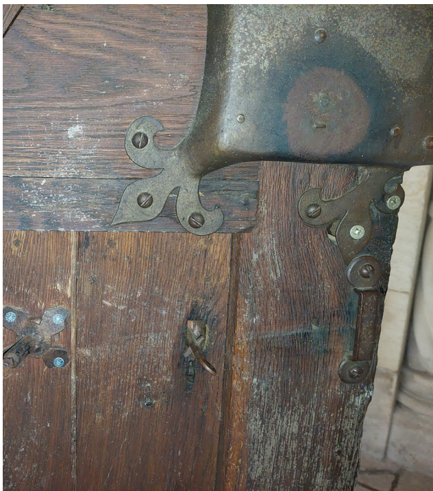
Serrurerie - Grossières réparations 6
